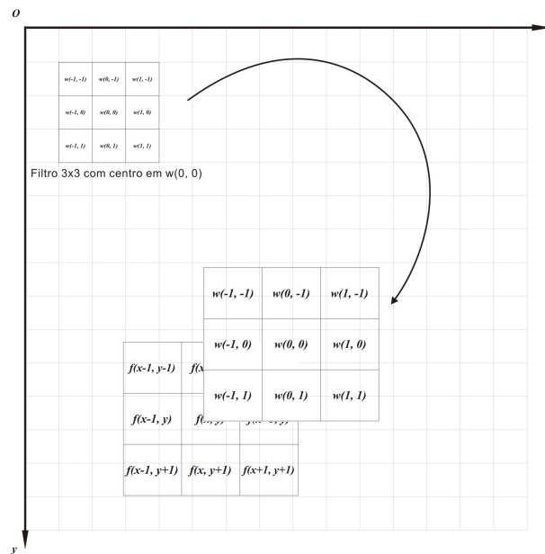
Figura 3: Aplicação de um filtro w de tamanho 3 \times 3 em uma imagem de entrada f . No detalhe, a sobreposição do filtro nos pixels correspondentes da imagem.
