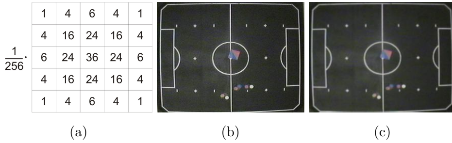
Figura 8: (a) filtro gaussiano 5x5. (b) imagem original. (c) imagem suavizada pelo filtro.
