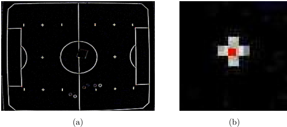
Figura 17: (a) Detecção das marcações do campo. (b) detalhe da marca do pênalti direito, o ponto destacado é a coordenada estimada pelo filtro de kalman.
