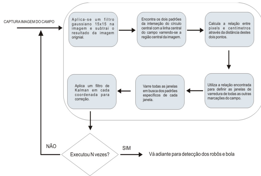
Figura 16: Fluxograma da aplicação do reconhecimento de padrões no campo.
