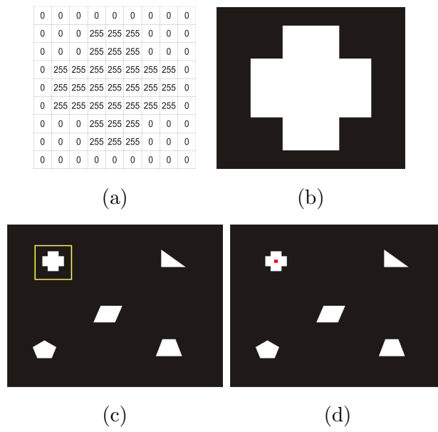
Figura 11: (a) subimagem p com o padrão. (b) marca de pênalti do campo. (c) detalhe da área que será varrida por p . (d) coordenada central do padrão encontrado.
