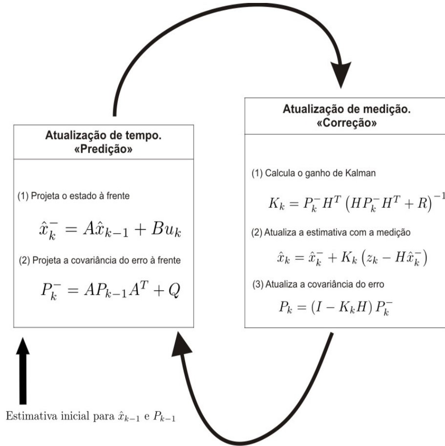
Figura 10: Diagrama da operação do filtro de Kalman (WELCH; BISHOP, 2001).
