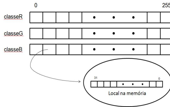
Figura 19: Vetores de classes de cores (KLANCAR et al., 2005). Cada classe de cor possui um bit que a representa dentre os 32 bits de cada posição nos vetores.
