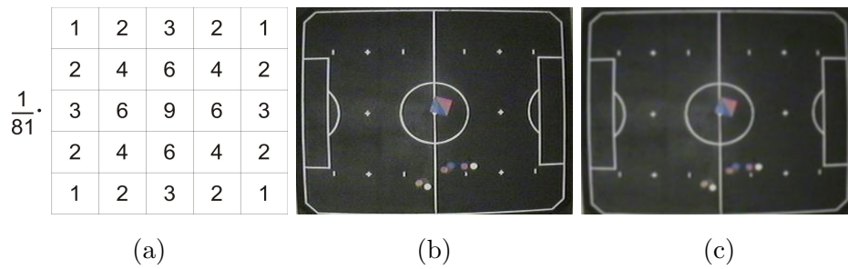
Figura 7: (a) filtro triangular 5x5. (b) imagem original. (c) imagem suavizada pelo filtro.
