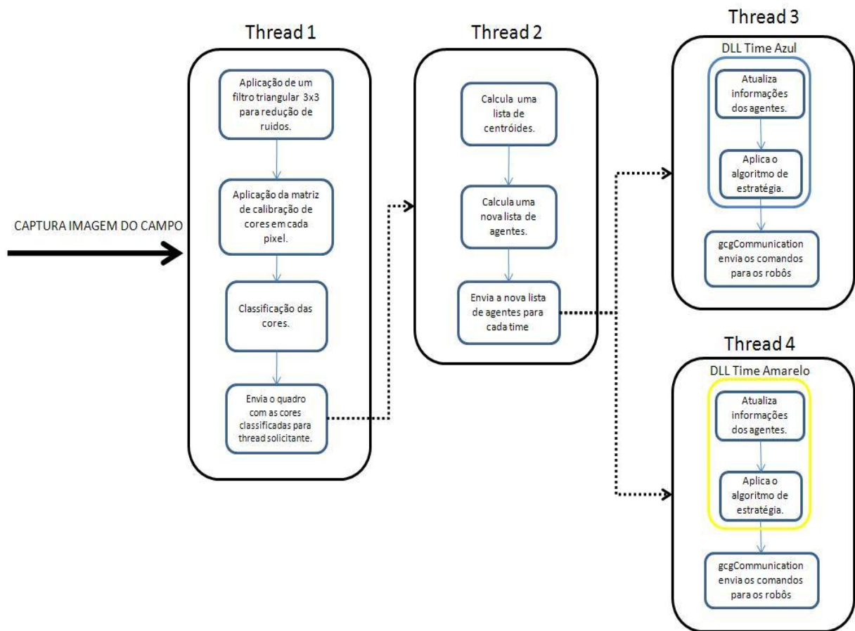
Figura 18: Fluxograma do funcionamento das threads.
