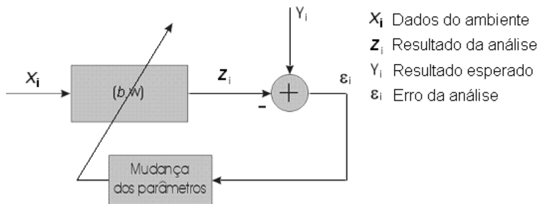
Figura 3-1 – Sistemas adaptativos
