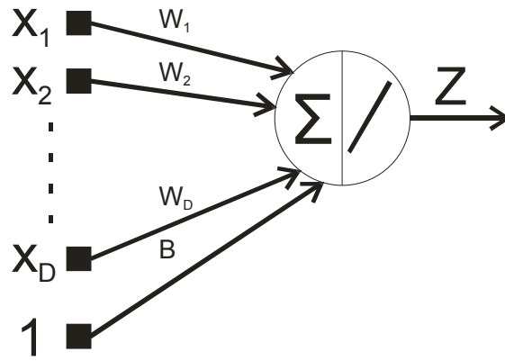
Figura 3-2 – Modelo Adaline
