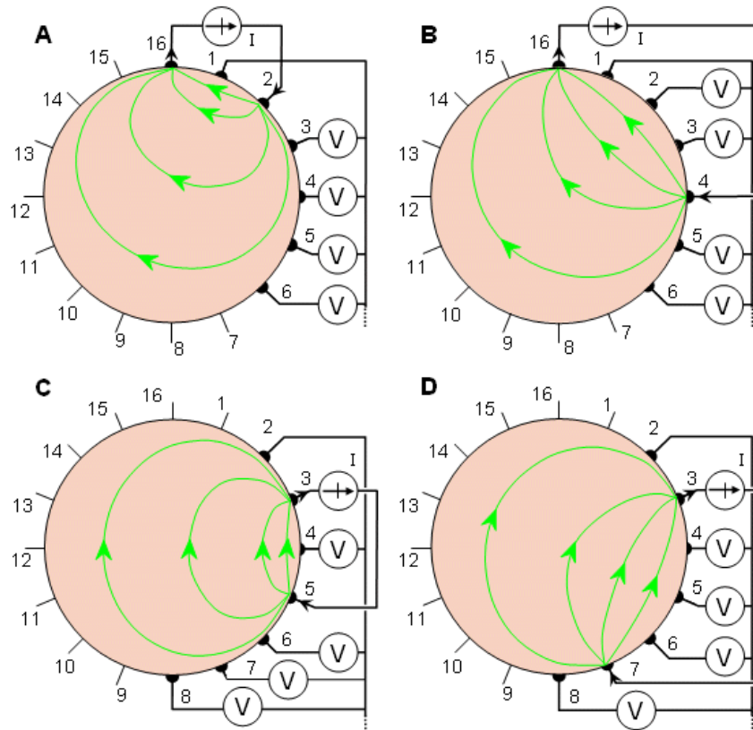
Figura 2.7: O método cruzado aplicado a um domínio de seção circular. São apresentados 4 casos de solicitação e as 4 primeiras medidas de diferença de potencial para cada caso. A imagem foi extraída de [58].
