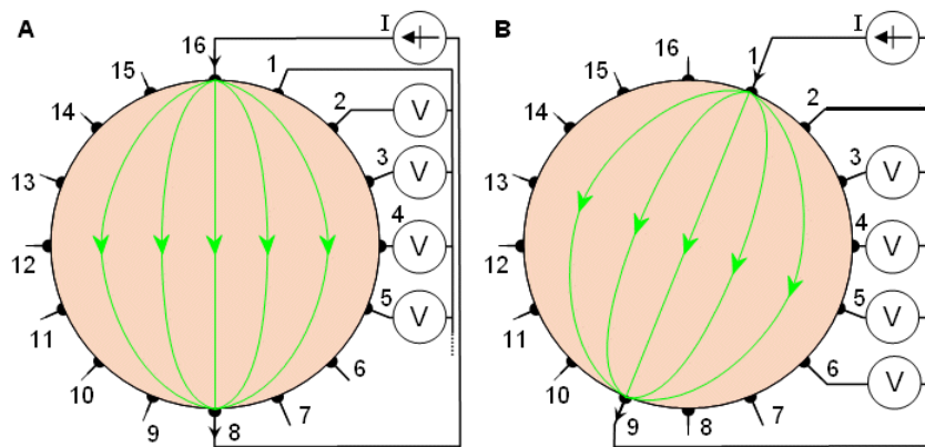
Figura 2.8: O método diametral aplicado a um domínio de seção circular. São apresentados 2 casos de solicitação e as 4 primeiras medidas de diferença de potencial para cada caso. A imagem foi extraída de [58].
