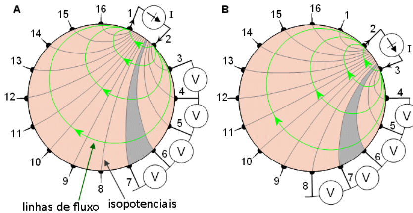
Figura 2.6: O método da vizinhança aplicado a um domínio de seção circular. São apresentados 2 casos de solicitação e 4 medidas de diferença de potencial para cada caso. A imagem foi adaptada de [58].
