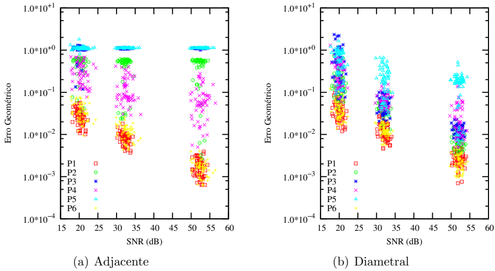
Figura 4.28: Relação entre SNR das medidas e erro geométrico.
