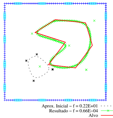
Figura 4.11: Identificação de inclusão com contorno não suave, a partir da mesma aproximação inicial usada no problema anterior. Ao final do procedimento, chega-se a 7 pontos de controle.
