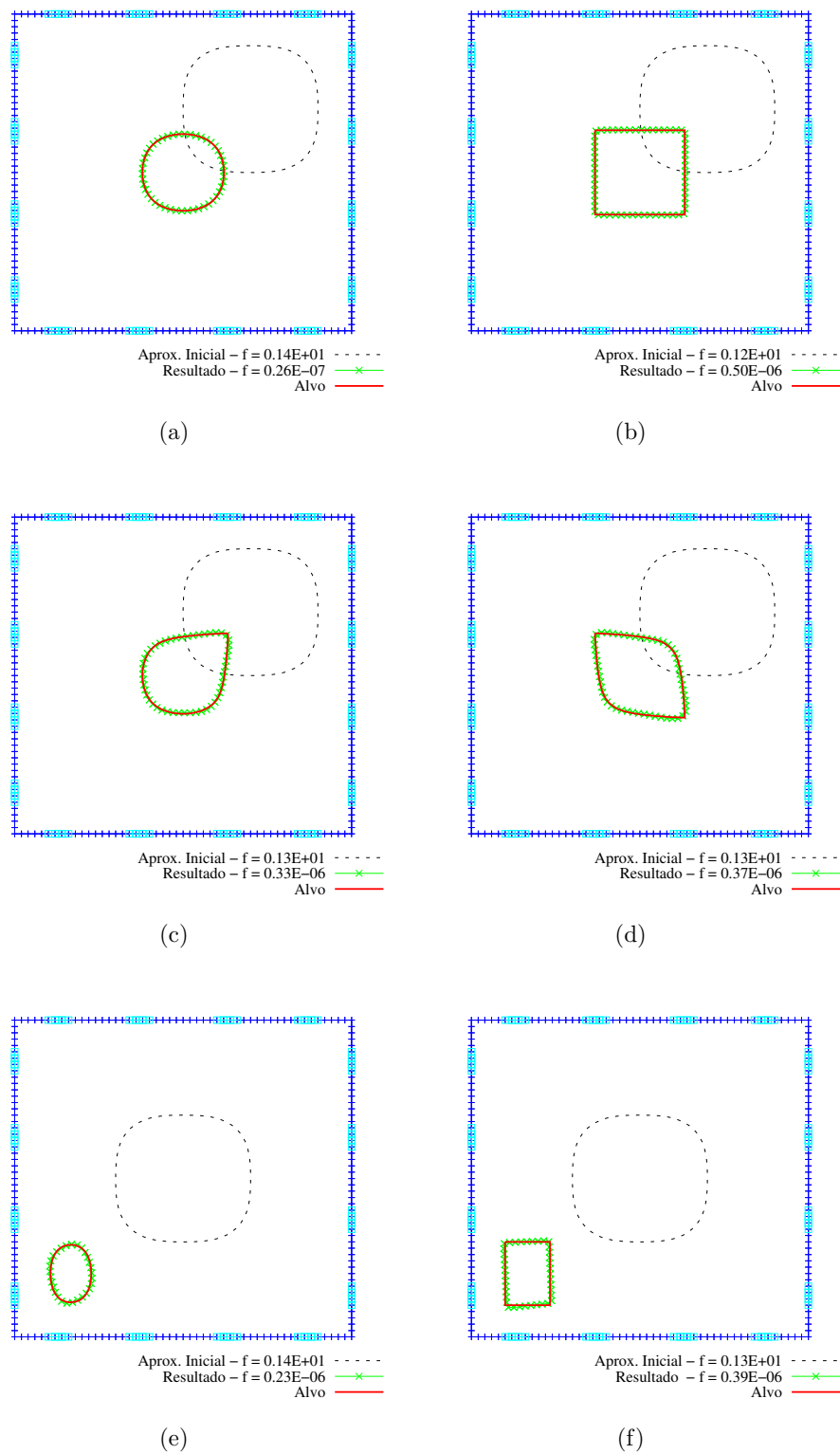
Figura 4.8: Identificação de 6 diferentes inclusões, algumas com formas suaves e outras angulosas.
