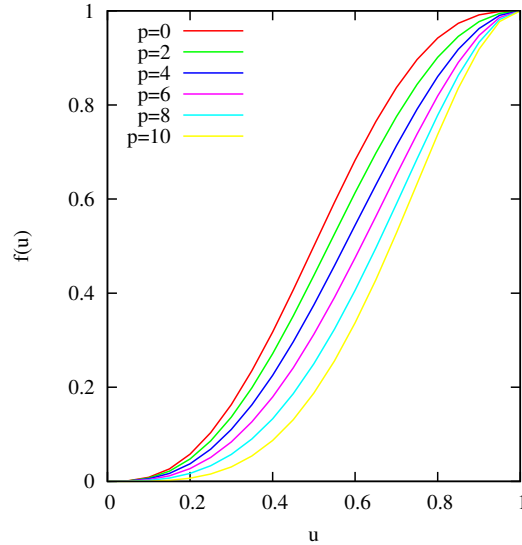
Figura 2.2: Polinômio f para alguns valores da constante p .
