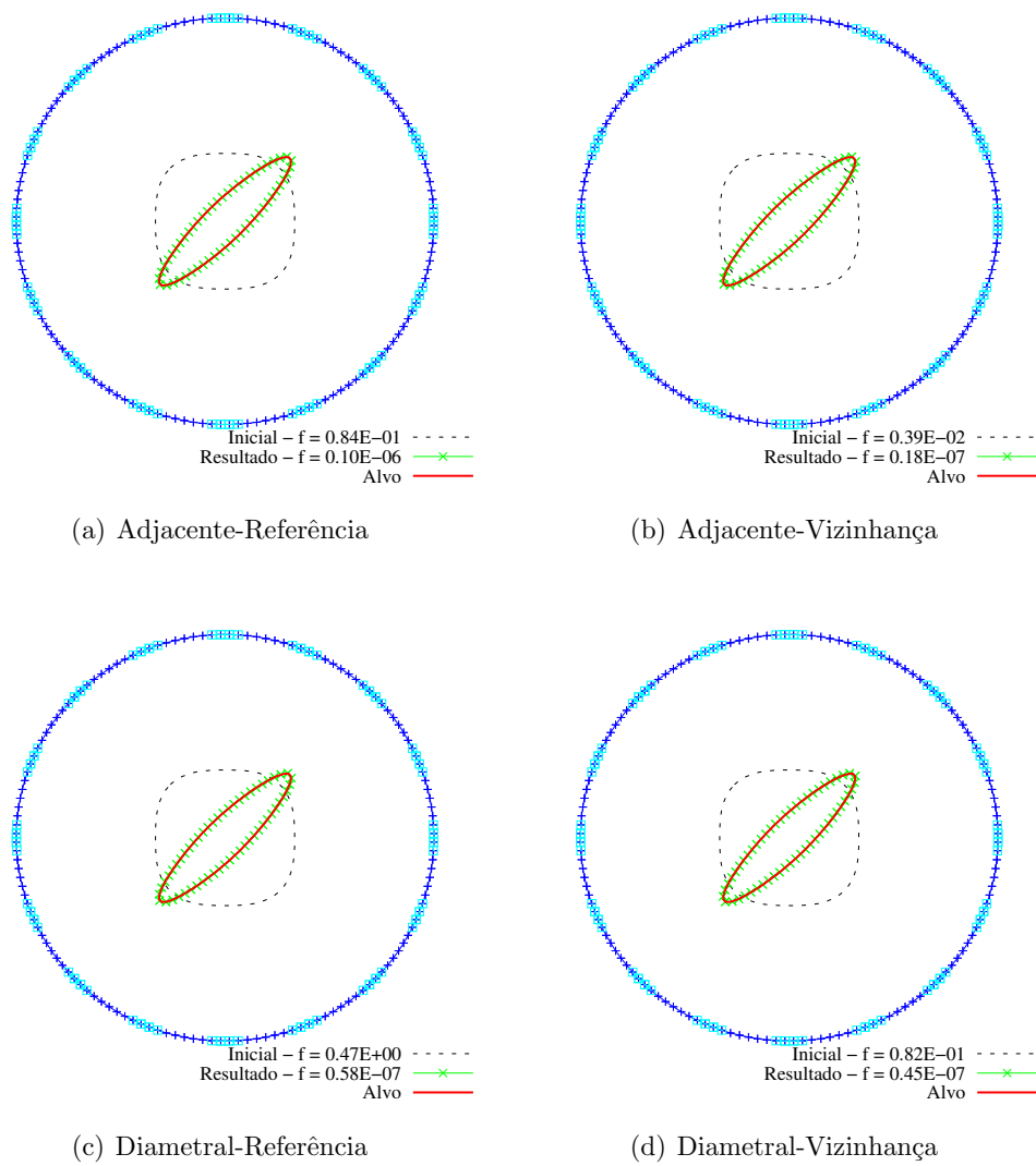
Figura 4.21: Comparação dos protocolos: Problema 1.
