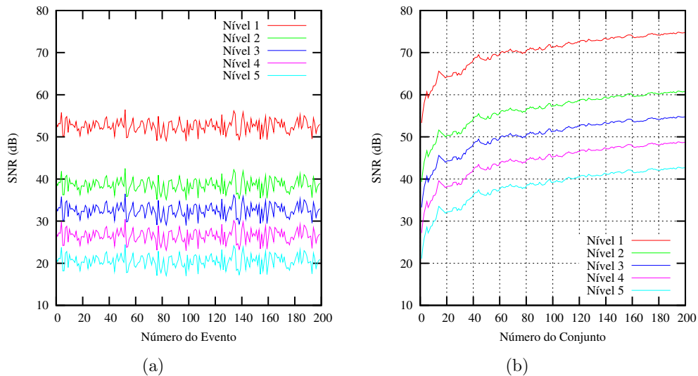
Figura 4.29: Protocolo Adjacente: (a) SNR do conjunto de medidas de cada evento de medição; (b) SNR de cada conjunto de medidas obtido pela média acumulada das medidas originais.
