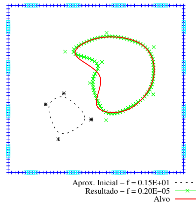
Figura 4.10: Identificação de inclusão a partir de spline com 4 pontos de controle, chegando a 7 pontos ao final do procedimento.
