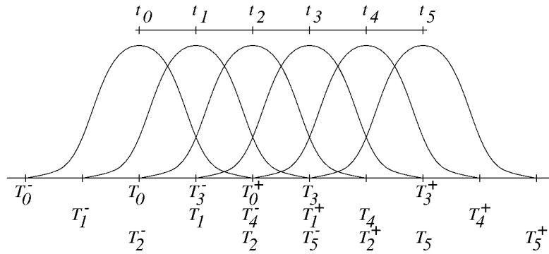
Figura 2.1: Funções de interpolação F_k(t) das X-Splines , extraída de [51].
