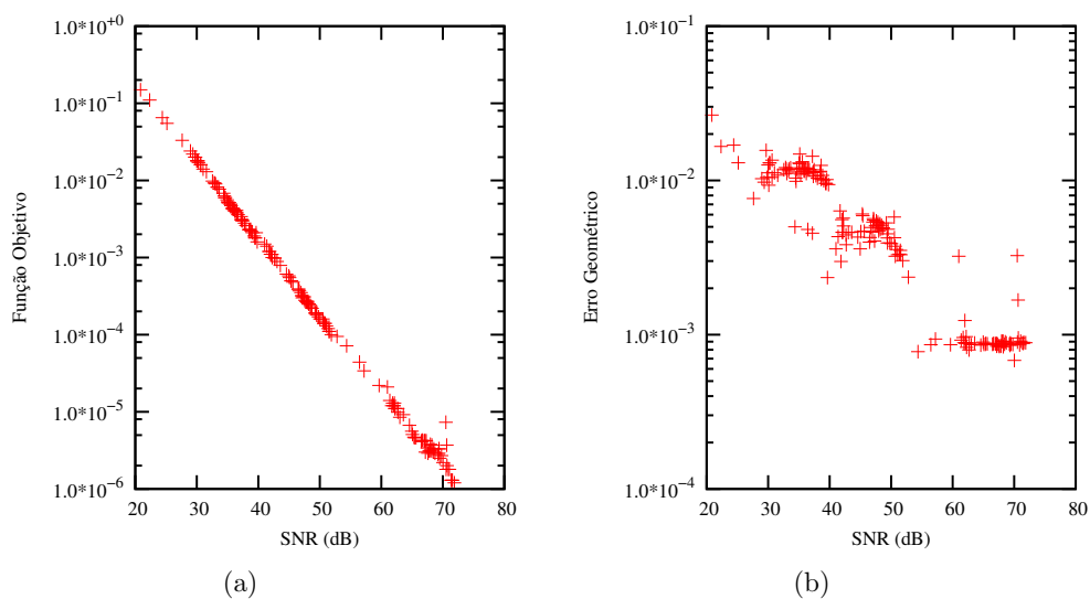
Figura 4.17: Relação entre o SNR de cada conjunto de medidas e o respectivo valor alcançado para a função objetivo (a) e o erro geométrico relativo de cada solução (b).
