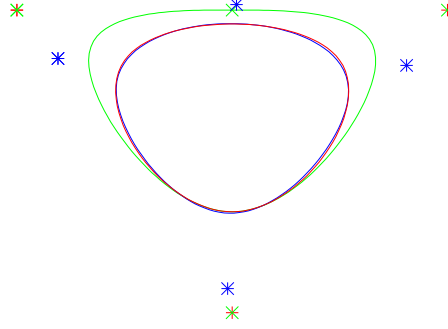
Figura 2.4: Comparação entre a spline original com 3 pontos de controle (vermelho) e curvas com 4 pontos de controle, antes da otimização (verde) e ao final do processo (azul). Os pontos de controle de cada curva são apresentados.
