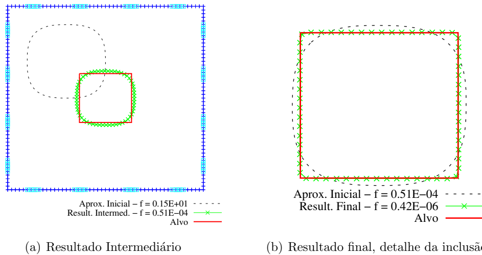
Figura 4.7: Resultado de cada etapa da minimização. Deve-se destacar que a inclusão resultante da primeira etapa, apresentada em (a), aparece como aproximação inicial da segunda etapa (b).
