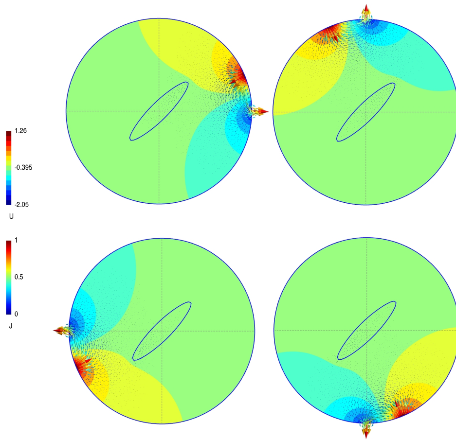
Figura 4.3: Distribuição do potencial ( U ) e da densidade de corrente ( J ) para os casos 1, 5, 9 e 13 de solicitação do protocolo adjacente em um domínio com uma inclusão posicionada no centro.
