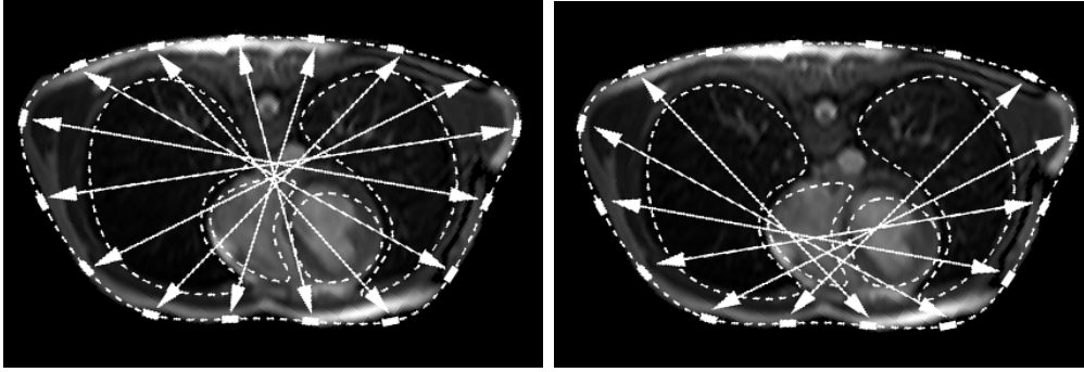
Figura 4.35: Estratégias para injeção de corrente elétrica: (a) Diametral e (b) Adaptada. As setas indicam os eletrodos utilizados para injetar e drenar corrente.
