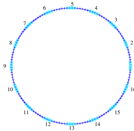
Figura 4.1: Domínio circular e distribuição dos 16 eletrodos no contorno externo.
