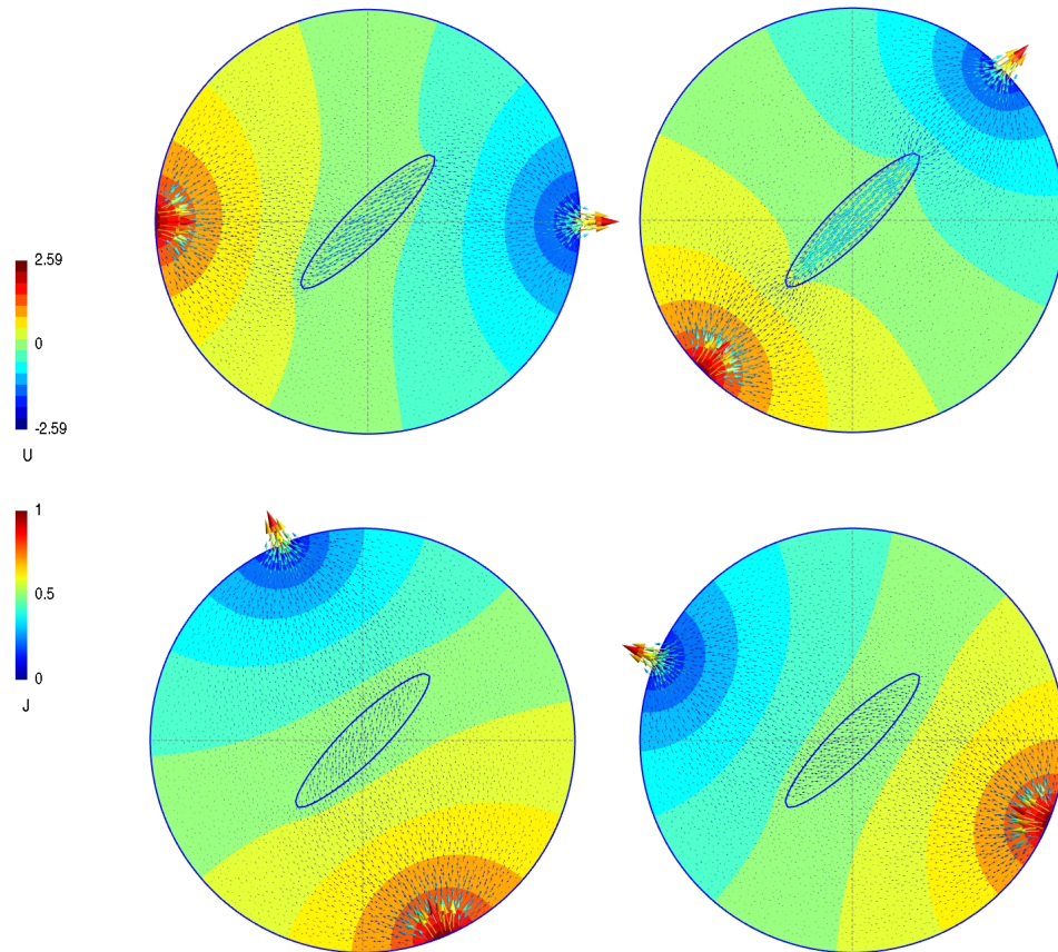
Figura 4.2: Distribuição do potencial (U) e da densidade de corrente (J) para os casos 1, 3, 6 e 8 de solicitação do protocolo diametral em um domínio com uma inclusão posicionada no centro.
