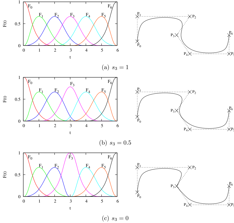
Figura 2.3: Influência do parâmetro s na curva resultante e nas funções de interpolação. Em todos os três casos foram usados: s_0 = 0 , s_1 = 1 , s_2 = 1 , s_4 = 1 , s_5 = 1 , s_6 = 0 . O parâmetro s_3 é diferente para cada caso.
