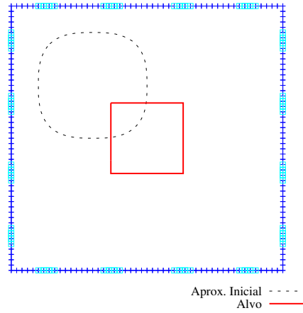
Figura 4.4: Inclusão para a qual foram geradas medidas de potencial no contorno e aproximação inicial para a qual foram calculados os erros relativos E_j .
