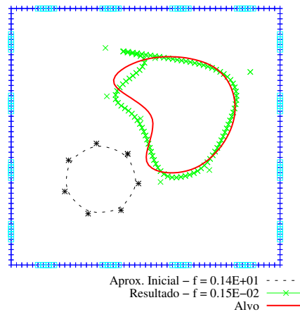
Figura 4.9: Identificação de inclusão a partir de spline com 7 pontos de controle.
