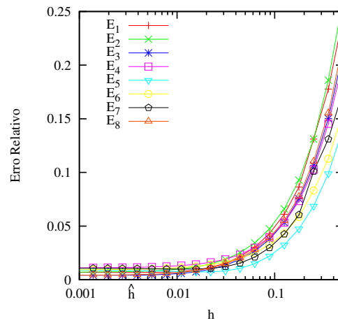
Figura 4.5: Influência do parâmetro h no erro relativo entre as derivadas obtidas por diferenças finitas e método semi-analítico.
