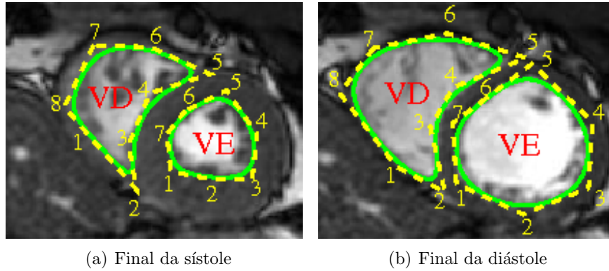
Figura 4.31: Imagens de Ressonância Magnética com a região de interesse delimitada pelas splines , em linha contínua. Poligonal em linha tracejada une os pontos de controle, numerados.
