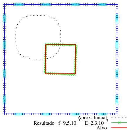
(a) 1º Conjunto
