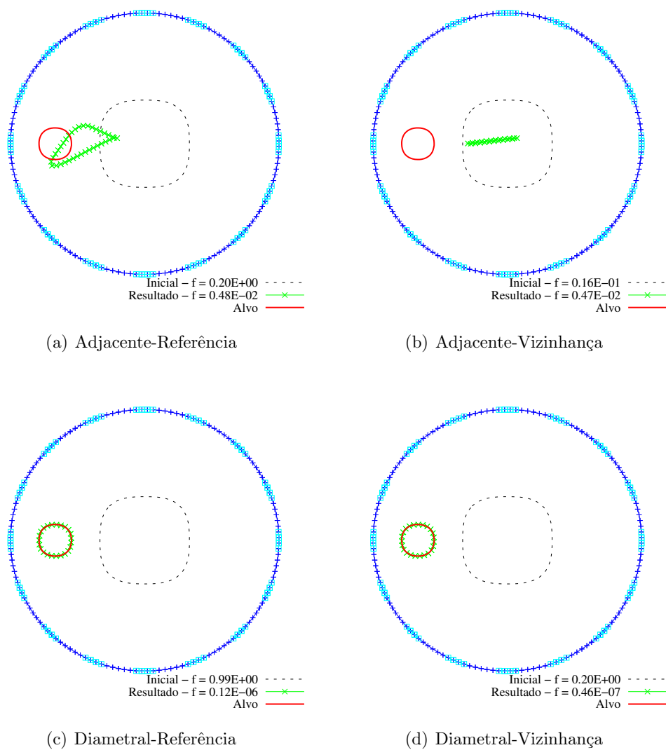
Figura 4.22: Comparação dos protocolos: Problema 2.
