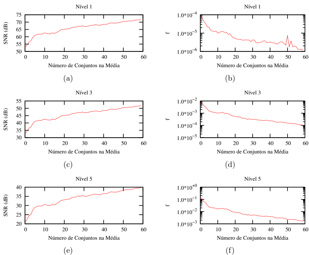
Figura 4.16: À esquerda os gráficos do valor do SNR referente a cada novo conjunto de medidas e à direita o valor da função objetivo que cada novo conjunto de medidas originou após a solução do problema inverso.
