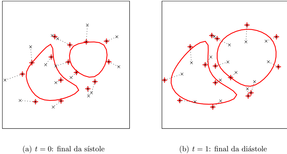
Figura 4.32: Comparação entre as curvas que contornam os ventrículos para valores extremos de t na parametrização com um único parâmetro. Em cada figura, os pontos destacados com uma cruz definem as curvas apresentadas.
