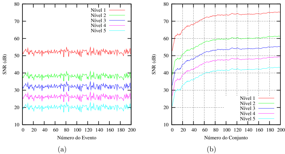
Figura 4.30: Protocolo Diametral: (a) SNR do conjunto de medidas de cada evento de medição; (b) SNR de cada conjunto de medidas obtido pela média acumulada das medidas originais.
