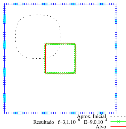
(c) Média com 40 conjuntos
