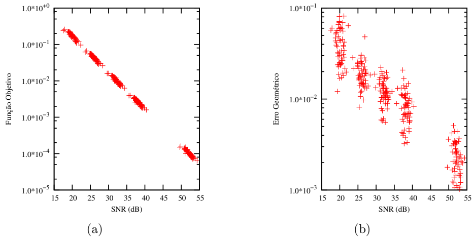
Figura 4.13: Relação entre o SNR de cada evento e o valor final da função objetivo (a) ou o valor do erro geométrico da identificação (b).
