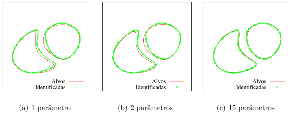
Figura 4.36: Resultados para o problema da identificação das cavidades ventriculares utilizando o protocolo adaptado de injeção de corrente. É possível comparar os resultados da otimização com 1, 2 e 15 variáveis de otimização.
