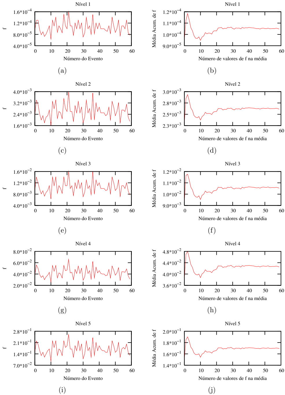
Figura 4.12: À esquerda são apresentados os valores da função objetivo ao final do processo de otimização para cada evento. À direita, apresenta-se a média acumulada do valor final da função objetivo, sendo que o eixo horizontal indica o número de valores da função objetivo que foram considerados na média.
