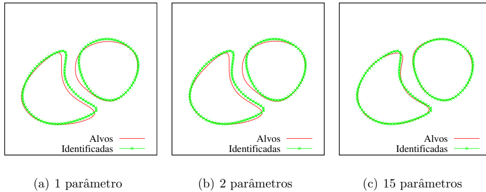
Figura 4.37: Resultados para o problema da identificação das cavidades ventriculares utilizando o protocolo diametral. O procedimento de identificação foi feito com 1, 2 e 15 variáveis de otimização.
