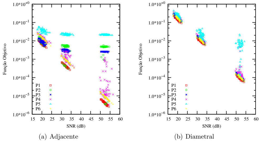
Figura 4.27: Relação entre SNR das medidas e valor alcançado da função objetivo.
