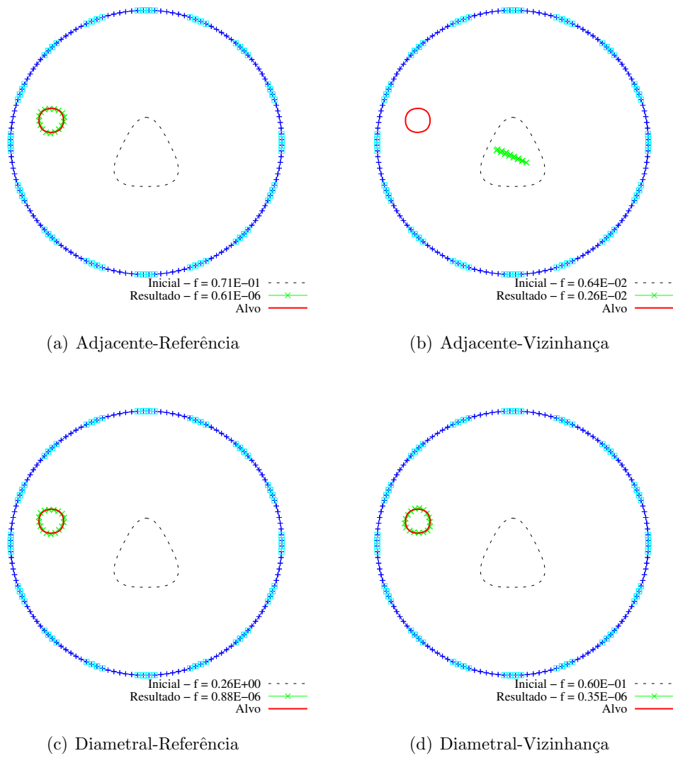
Figura 4.23: Comparação dos protocolos: Problema 3.
