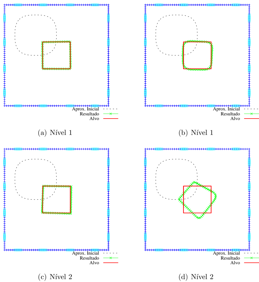
Figura 4.14: À esquerda são apresentados os melhores resultados e à direita os piores para os níveis 1 e 2 de ruído.
