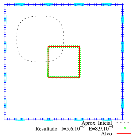
(b) Média com 20 conjuntos
