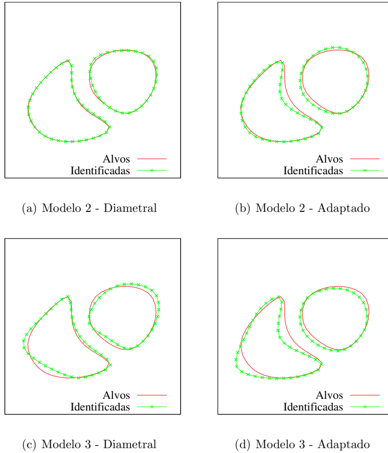
Figura 4.38: Resultados para o problema de identificação das cavidades ventriculares, considerando os modelos 2 e 3 de distribuição de condutividades e dois protocolos de injeção de corrente.
