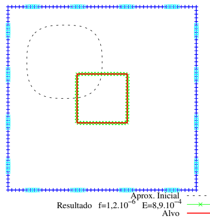
(d) Média com 60 conjuntos
