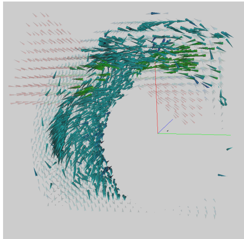
(a) Coloração dada por \mu_2
