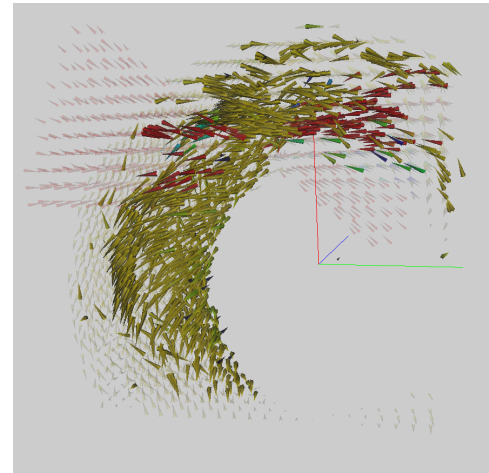
(b) Coloração dada por \Upsilon = \mu_2 + c_l
