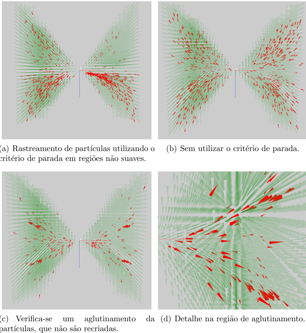
Figura 4.14: Análise do critério de parada das partículas (vermelho) em um campo tensorial elíptico(verde).
